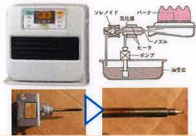
気化器のニードル部のタールも取れより完全燃焼に
